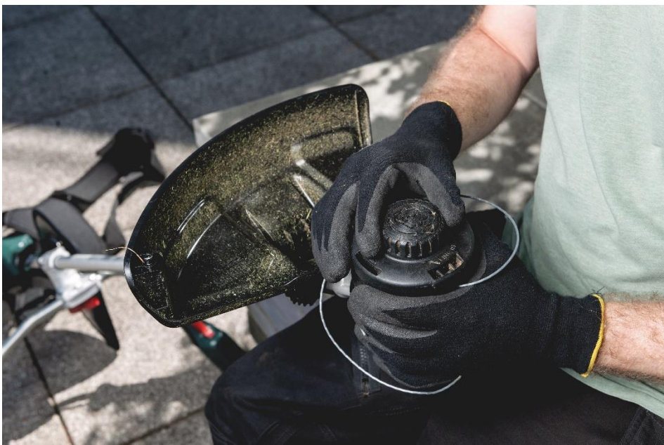
Schnell und werkzeuglos: Den Faden in den Metabo Freischneidern FSB 36-18 LTX BL 40 und FSD 36-18 LTX BL 40 wechseln Anwender ohne die Spule öffnen oder abnehmen zu müssen. Foto: Metabo
